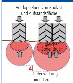
Grafik 3: DOPPELTE RADLAST – DOPPELTE AUFSTANDSFLÄCHE
