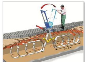
Spaltenbodenmischer Porco für Schweineställe, Torro für Rinderställe
